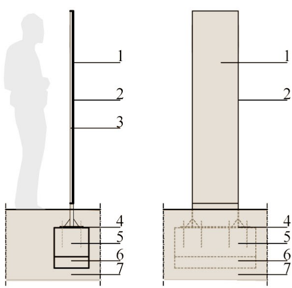
6. TOTEM INFORMATIVO_ SCALA 1:50
