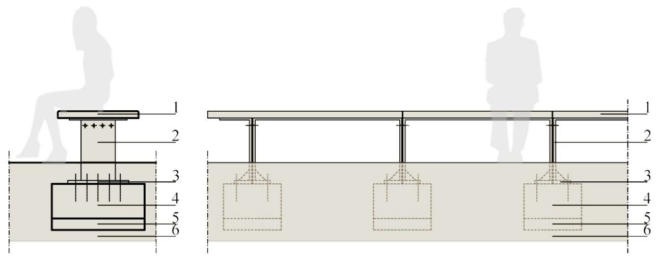
4. SEDUTA RETTILINEA_ SCALA 1:50
